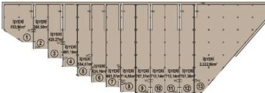
642 / 4 D BLOK ALT YOL KOTU KAT PLANI
