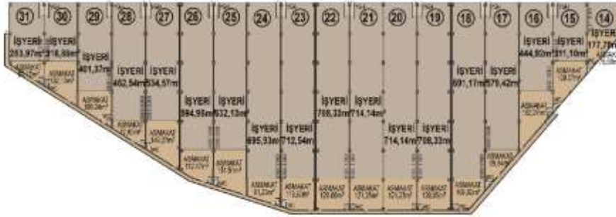
642 / 4 D BLOK ÜST YOL KOTU & ASMA KAT PLANI
